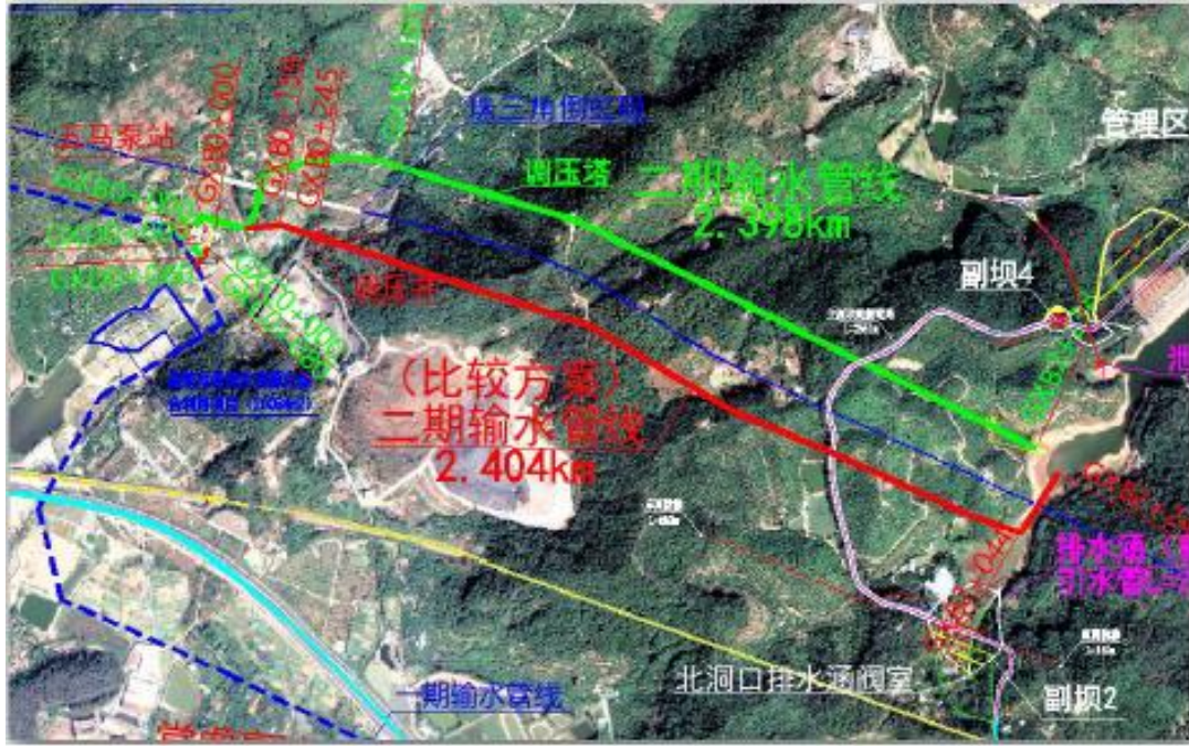
输水线路平面布置图
